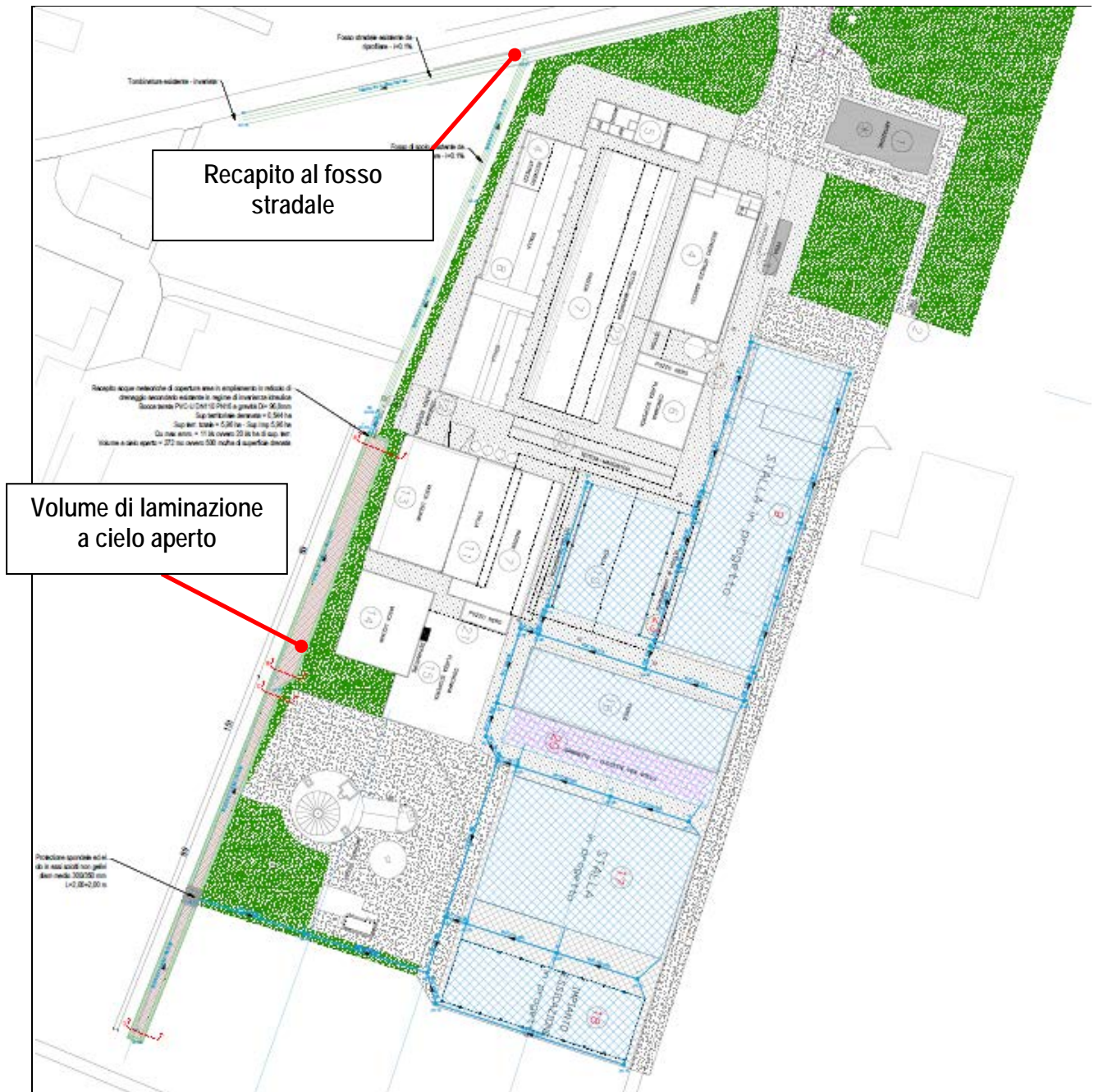
Figura 12: Caratteristiche dell'invaso di laminazione.
