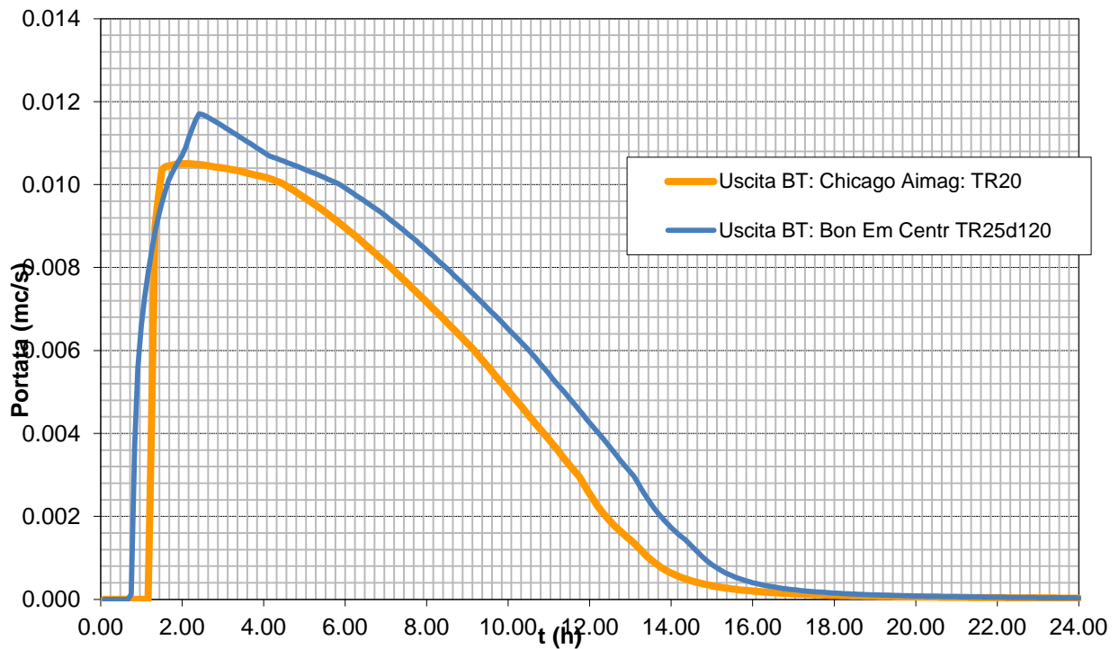
Grafico 3: Confronto tra idrogrammi in uscita dall'intero bacino drenato: ietogramma rettangolare Chicago Aimag Spa TR = 20 anni durata 4 ore e ietogramma rettangolare Bonifica Emilia Centrale TR = 25 anni durata 120 minuti.
