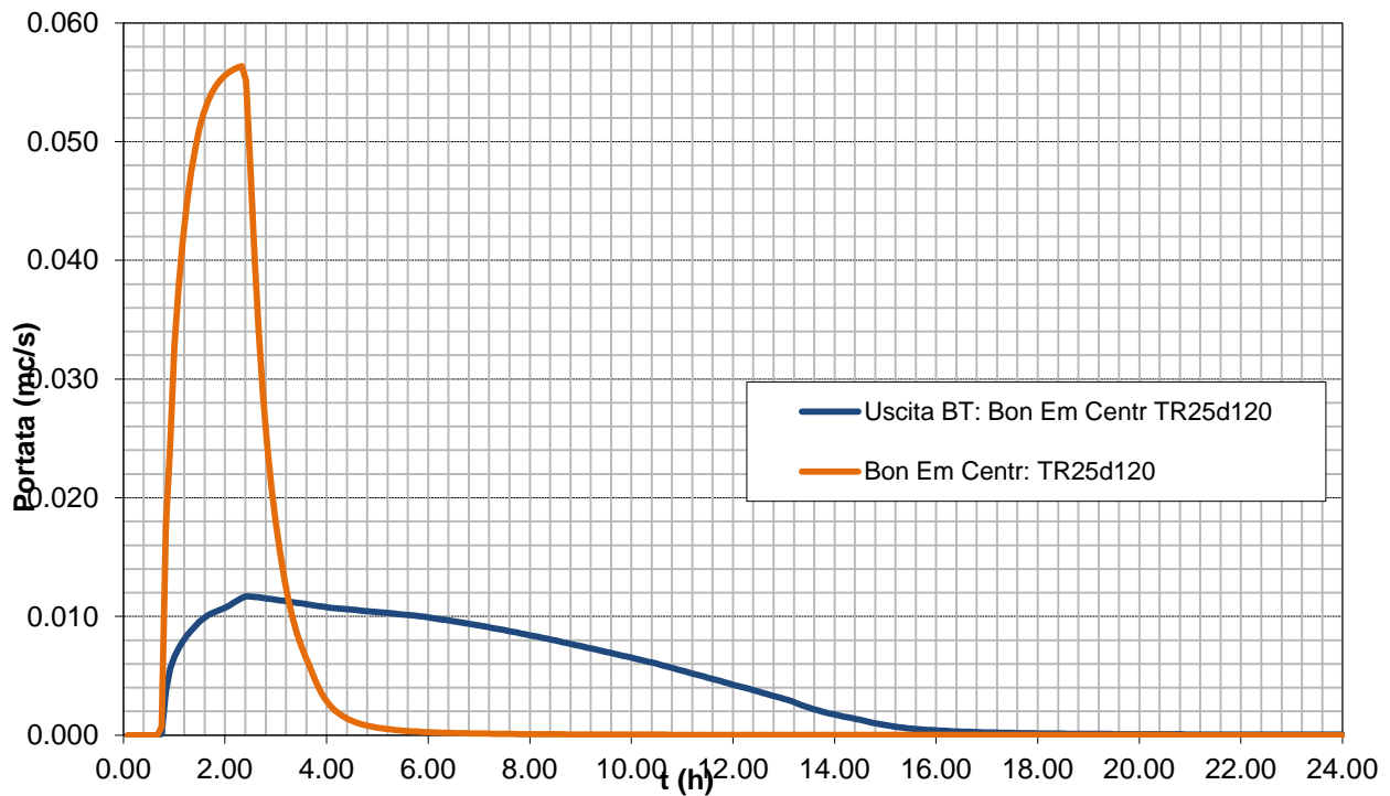
Grafico 2: Idrogrammi di piena caratteristici del lotto in esame calcolati in corrispondenza dell'immissione nel recapito (nodo 7) in assenza/presenza di regolazione della portata e vasca di laminazione – ietogramma rettangolare Bonifica Emilia Centrale TR = 25 anni durata 120 minuti.
