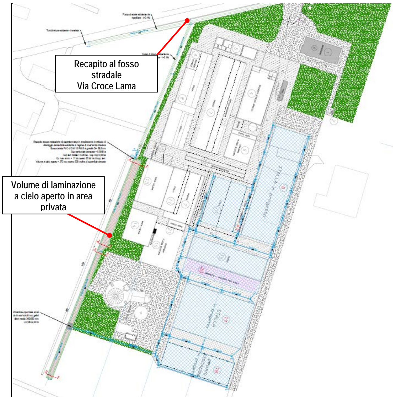
Figura 5: Planimetria generale della rete acque meteoriche di copertura interna al lotto.
